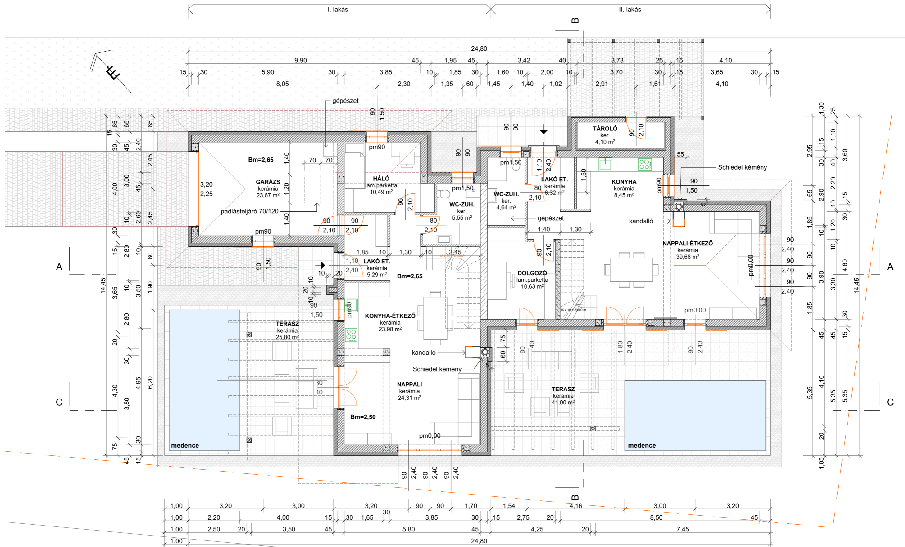
FÖLDSZINTI ALAPRAJZ
